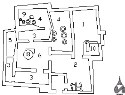
تصویر ۲۲. نقشه یک واحد مسکونی صنعتی در شهداد مأخذ: (بازترسیم از کیانی، ۱۳۶۶: ۷۲)
