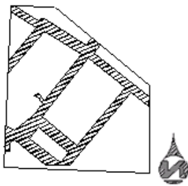
تصویر ۱۶. پلان بخش از روستای پیش از تاریخ قبرستان و نوع اتصالات در کنجها (مأخذ: بازترسیم از میراث فرهنگی قزوین)
